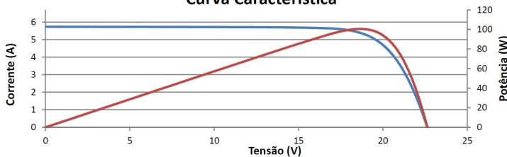
Curva Característica
